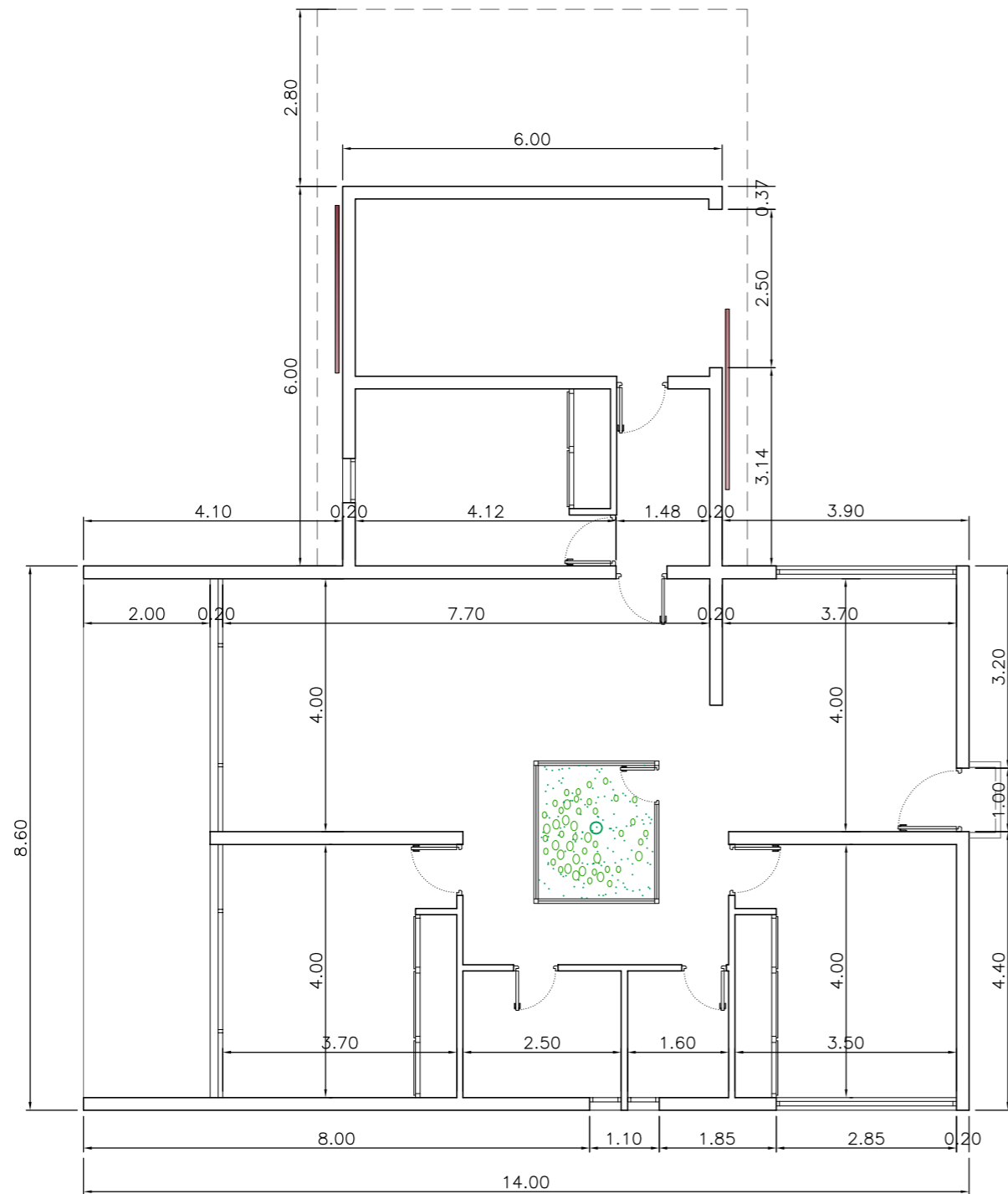
PLANTA BAJA - COTAS
