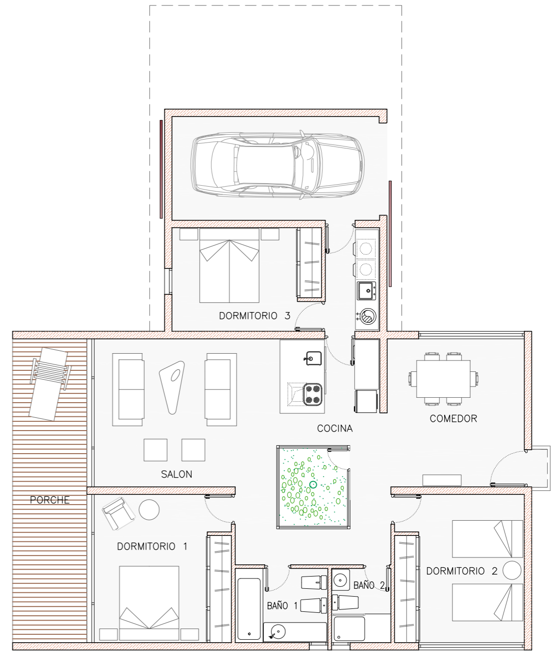
PLANTA BAJA - USOS
