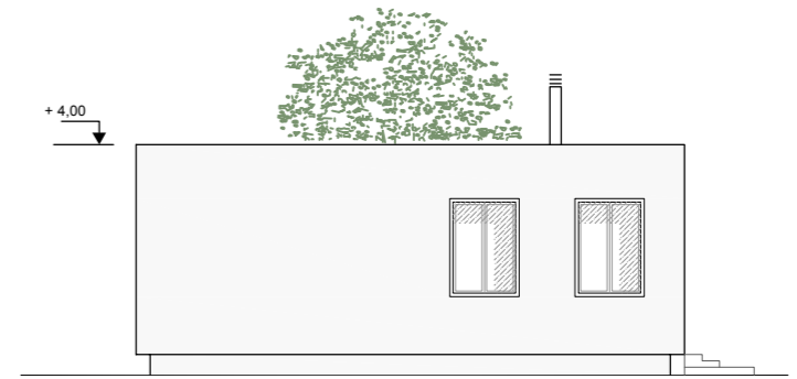
ALZADO LAT. IZQUIERDO
