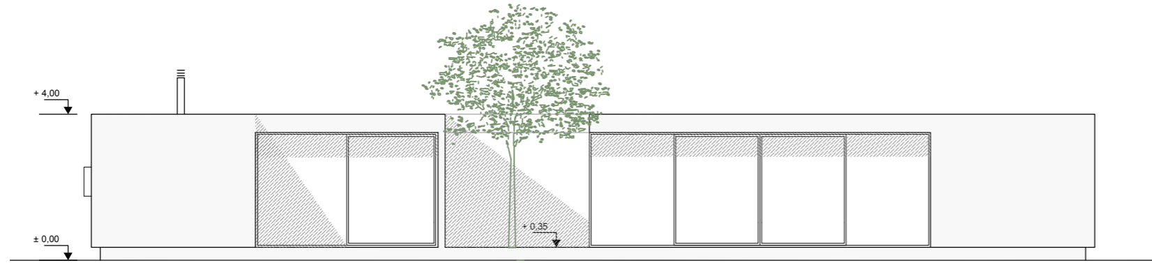
ALZADO POSTERIOR
